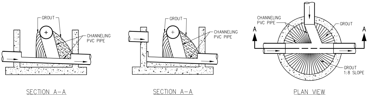
SECTION A-A
